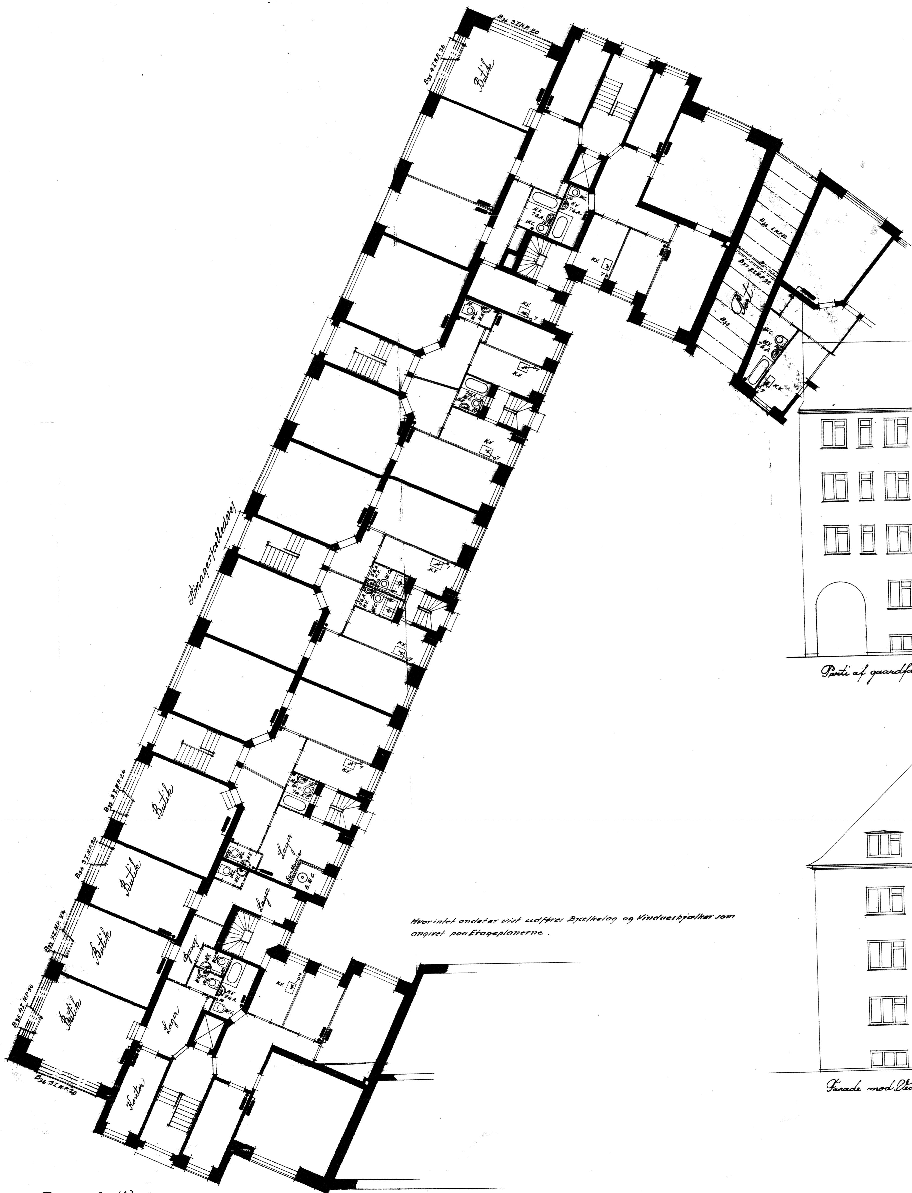
Parti af stueplan.
